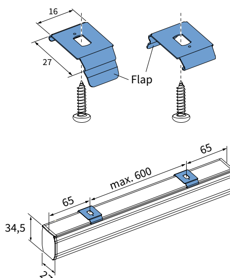
Profiel 27 [mm] x 34,5 [mm] Clip
